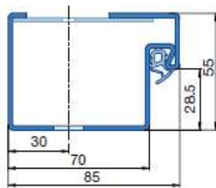
Blockzarge für den Einbau auf der Wand
